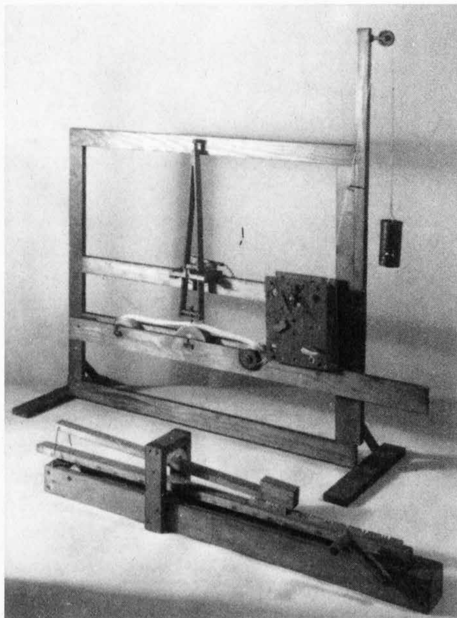
Geber (vorne) und Empfänger (hinten) des ersten Schreibtelegraphen mit Gewichtsantrieb von Samuel Morse, 1837; Abbildung aus: Meyers Enzyklopädisches Lexikon, Bd. 23, Mannheim/Wien/Zürich 1978, S. 295.
