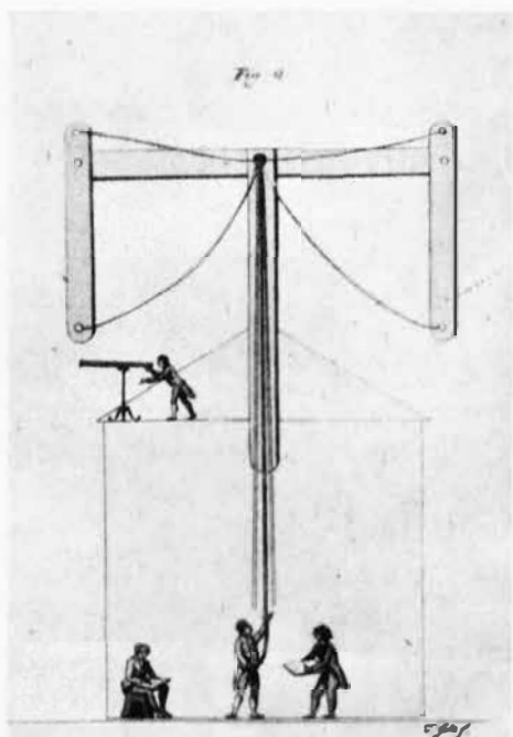
Französischer optischer Telegraph 1794-1853, Station auf dem Louvre, um 1800; Abbildung aus: Pieper, Geschichte (wie Anm. 1), S. 42.
