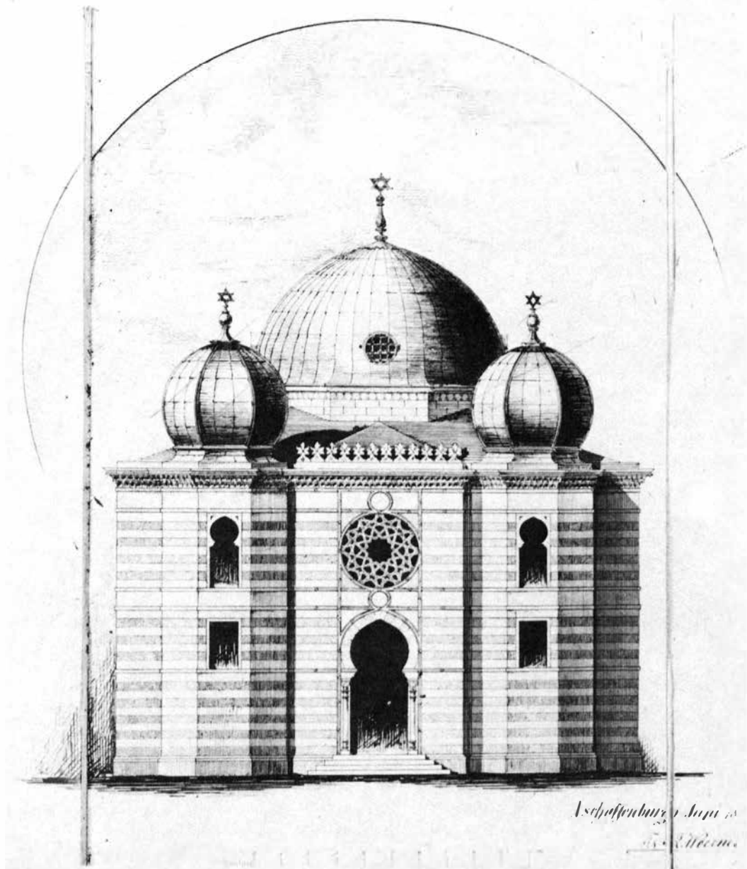
Fassadenentwurf zum Neubau der Synagoge an der Entengasse 1891/93
